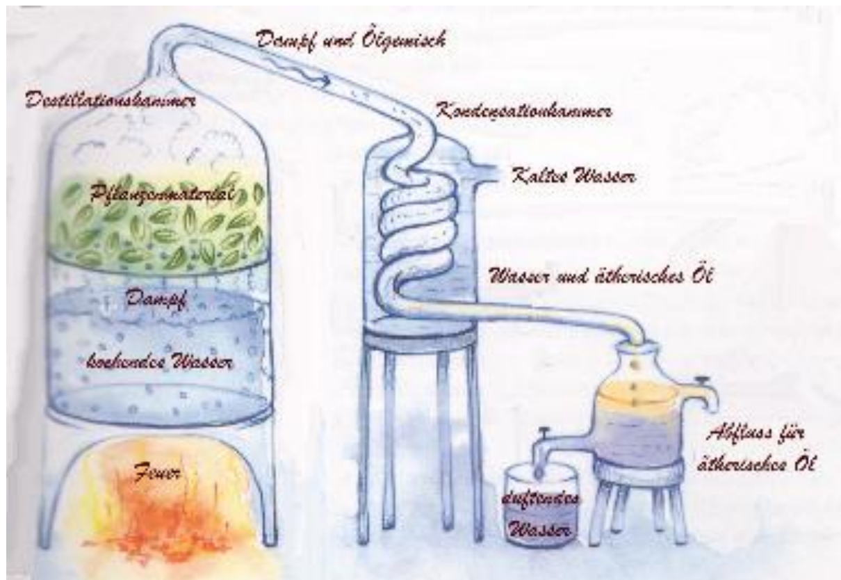
Abbildung 10: Destillationsprozess
